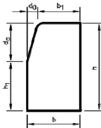
DIBUJO 1: Dimensiones y tolerancias. Bordillo y pieza complementaria rígola de hormigón (cm)
