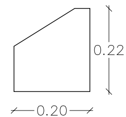
BORDILLO EN ACERAS Escala. 1:10
