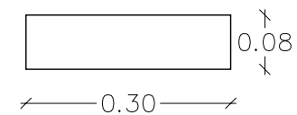
BORDILLO EN ACERA-JARDIN Escala. 1:10
