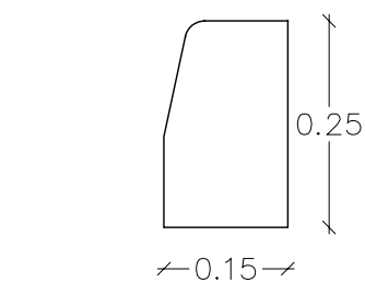
BORDILLO EN VIALES Escala. 1:10
